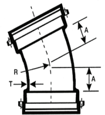
PO x PO Bend 22-1/2°
