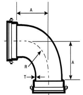
PO x PO Bend 90°
